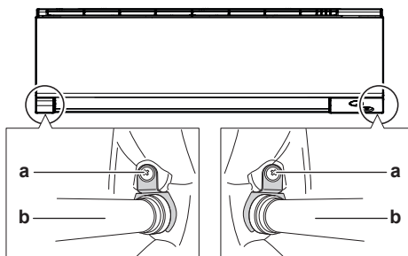
a Zavrtanj za fiksiranje izolacije b Odvodno crevo
