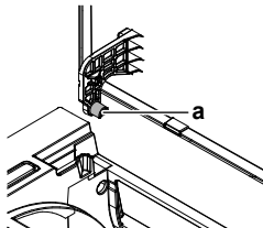
a Osovina prednje ploče
