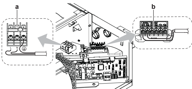
a Terminalni blok napajanja b Terminalni blok korisničkog interfejsa
